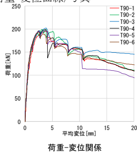
荷重-変位関係
