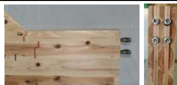
ラミナの局所的な引張破壊
