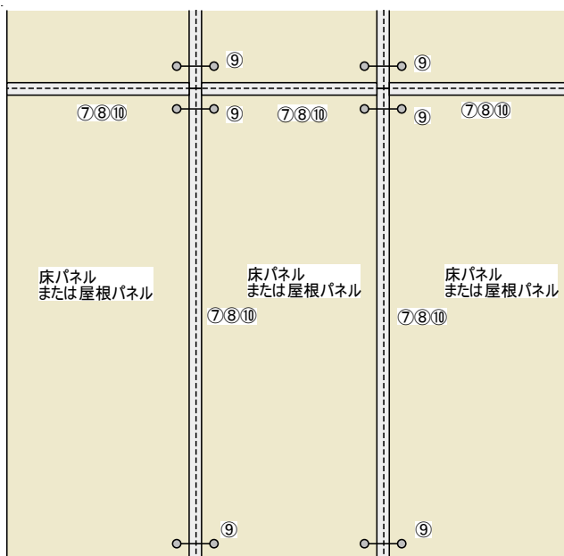
< 水平構面 >
