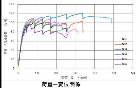
荷重-変位関係
