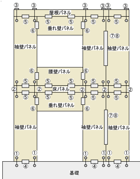
< 鉛直構面 >
