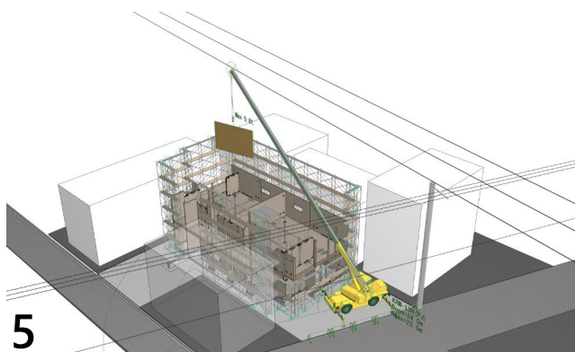
5. 2FCLT壁パネル吊り込み
